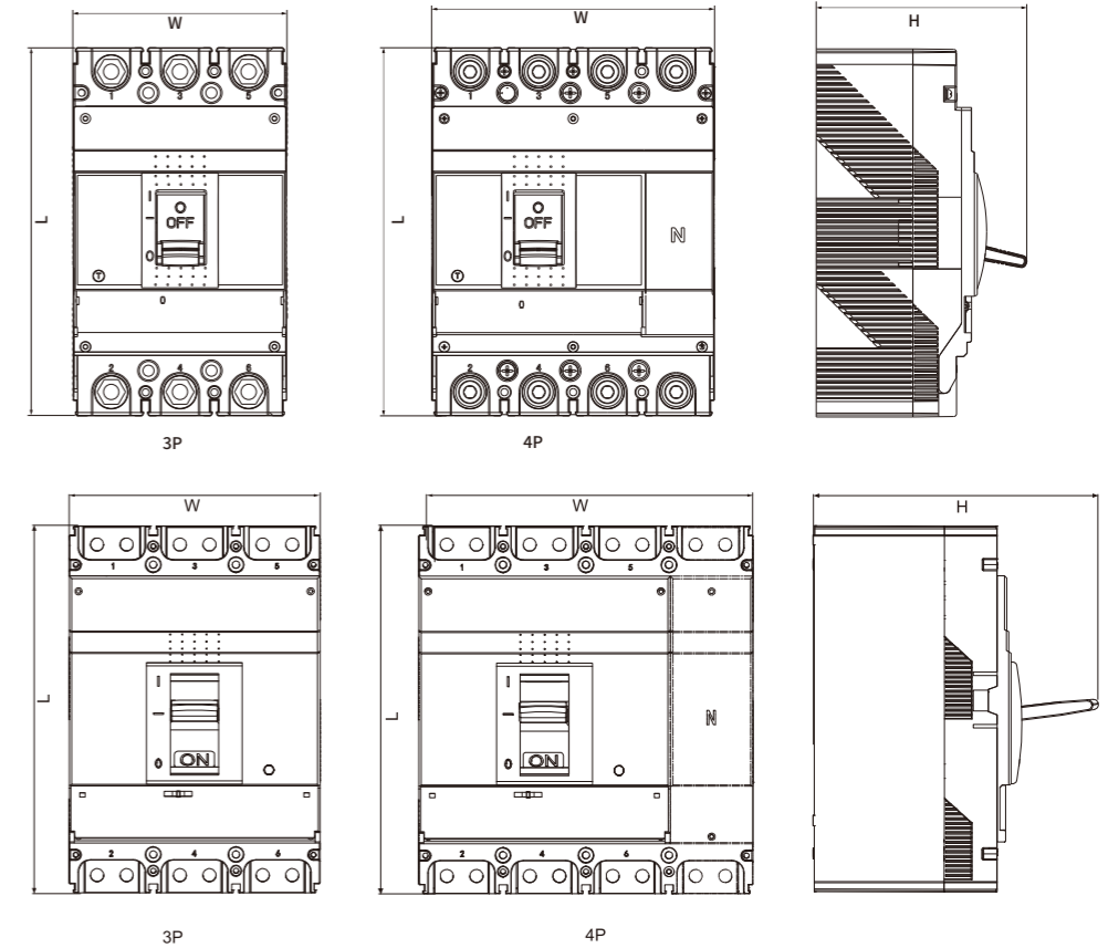
SGM6 Dimensions mm(L×W×H)
