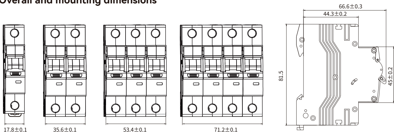
SGR-63M-DC
